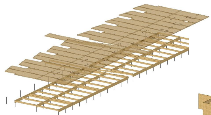
Paneles contralaminados de clt sobre estructura de madera laminada.
