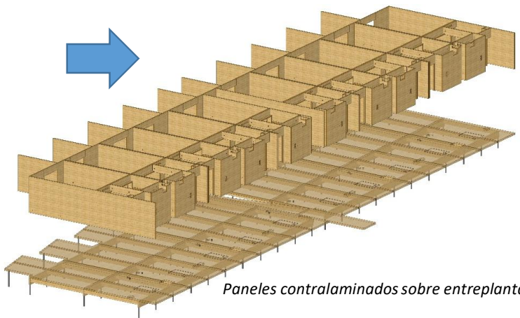
Paneles contralaminados de clt sobre estructura de madera laminada.
