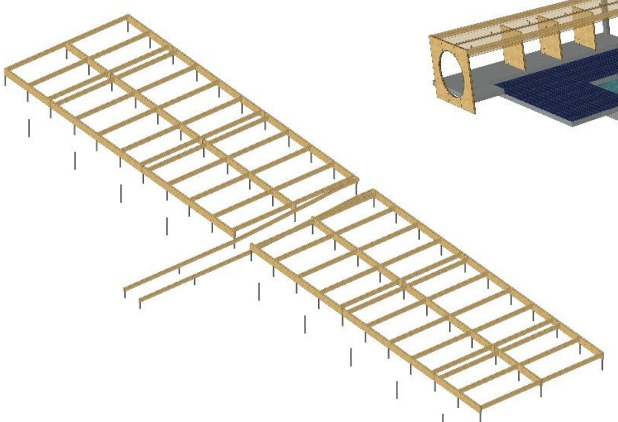
Estructura madera laminada GI 24h de pino radiata sobre micro-pilotes metálicos para arrancar la estructura del hotel Lamintin a Senegal.
