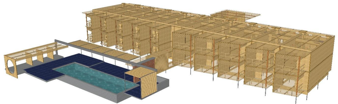
Paneles contralaminados sobre entreplanta
